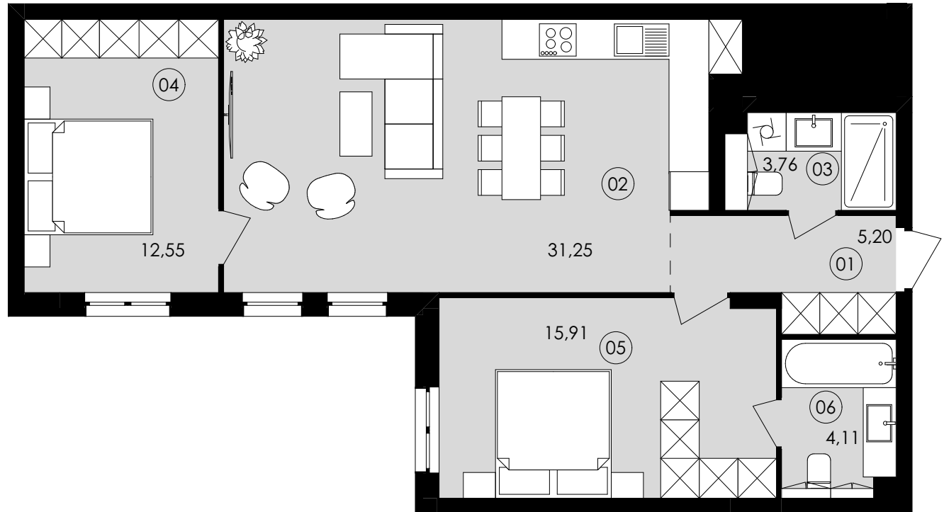
Експлікація приміщень
